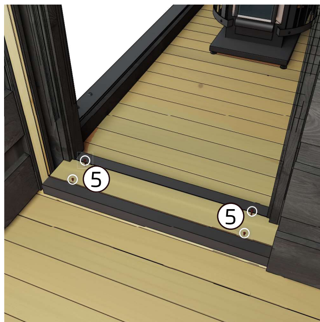
11. Fixez la planche de seuil à l'aide des vis ( 5 ). Des trous sont déjà pré-perçés dans la planche de seuil.
