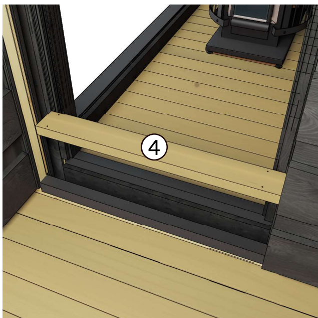
10. Asettele astinlauta ( 4 ) saunan ja pukuhuoneen väliin.
