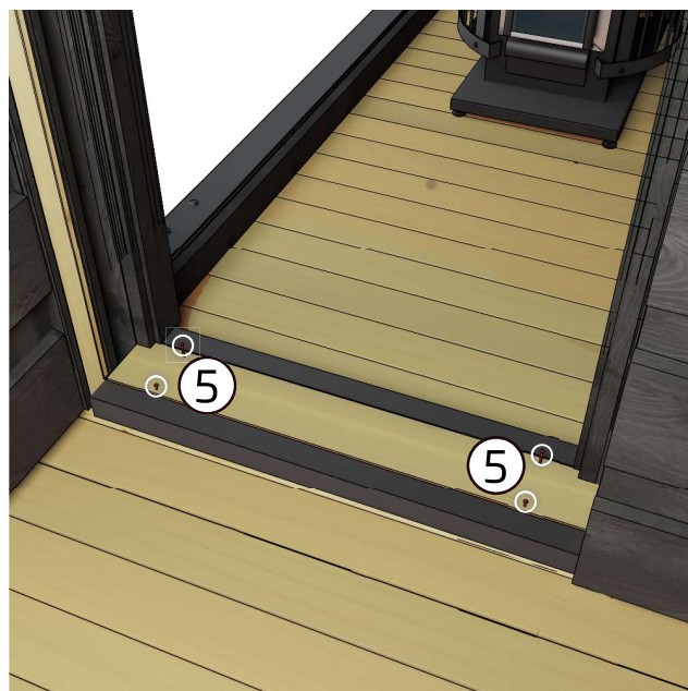
11. Bevestig de drempel met schroeven ( 5 ). De drempel heeft voorgeboorde gaten.
